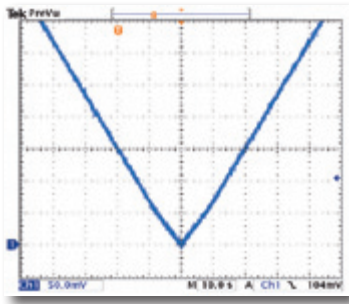
模拟电池缓降及缓升供压试验
