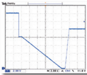
模拟电池供压瞬降试验
