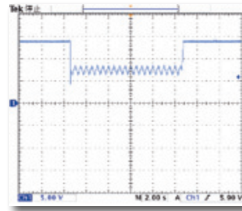
ISO 16750-2启动电压曲线试验
