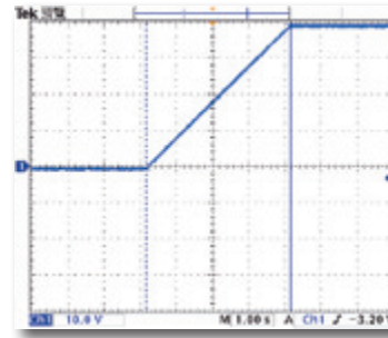
输出电压爬升斜率控制
